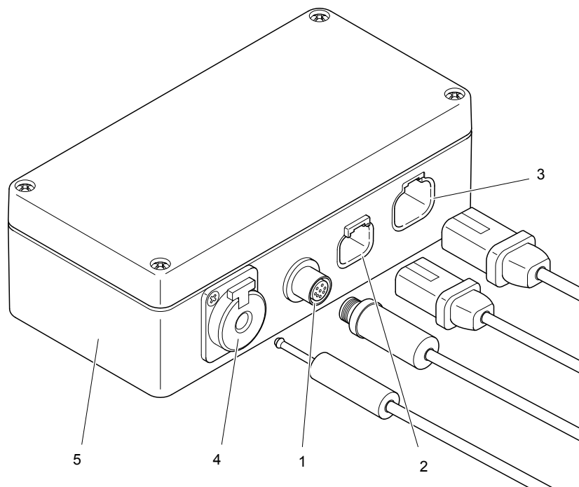
Abb. 5 Funkmodul
