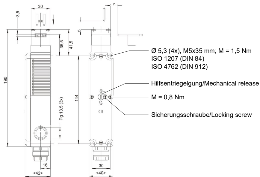
Fig. 1 Maßzeichnung/Dimensional drawing
