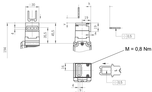
Fig. 3 Betätigungskopf mit Einführtrichter/ Actuator head with insertion funnel
